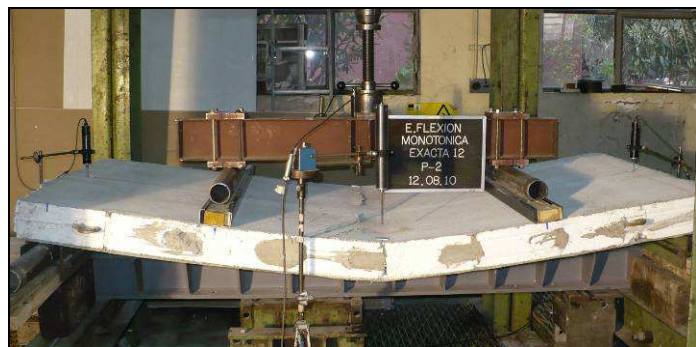
Fotos 6 y 7. Modo de falla de la muestra N° 2.
