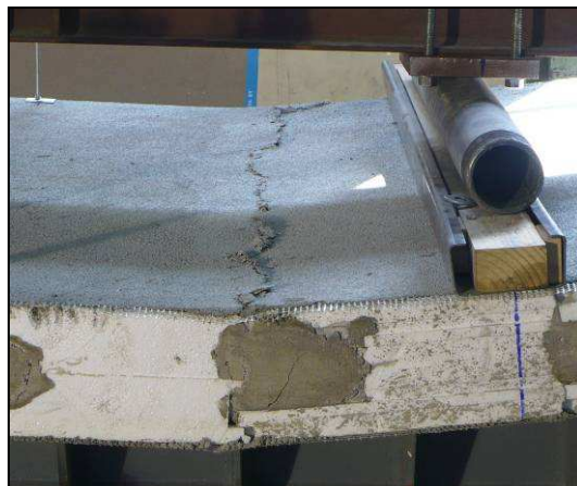
Fotos 4 y 5. Modo de falla de la muestra N° 1.
