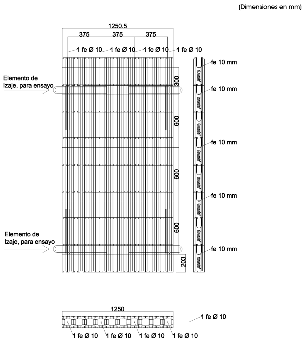
Figura 2: Esquema de muestra de ensayo, muro "Exacta 12".
