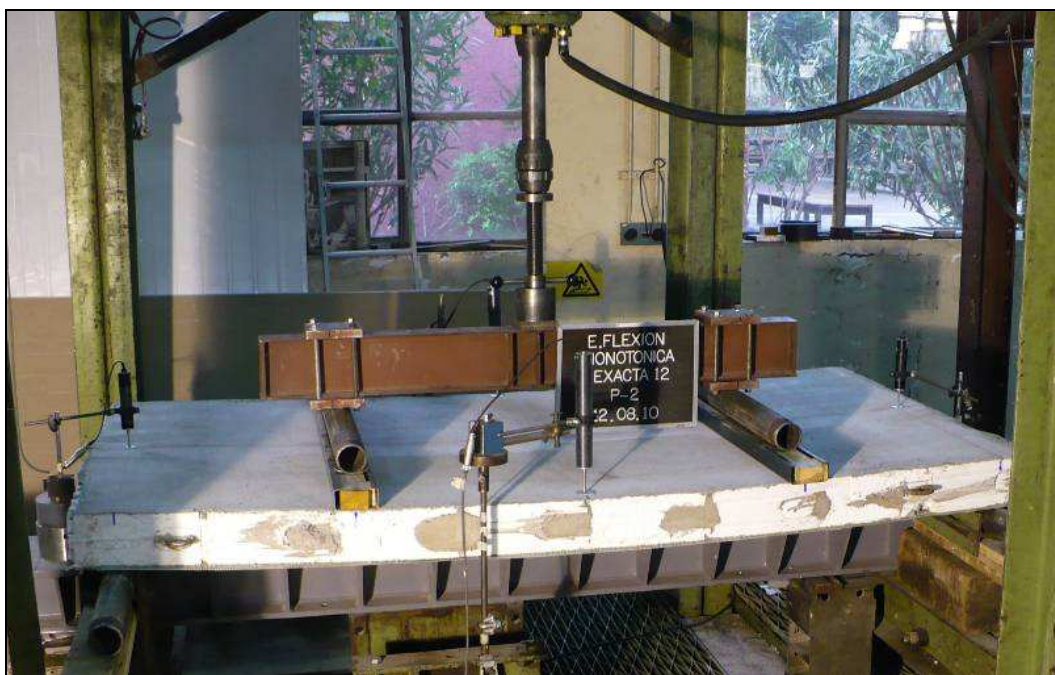
Foto 3. Vista general del montaje del ensayo de flexión al muro.
