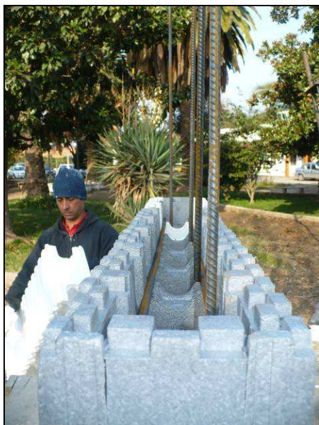
Foto 1. Construcción de probetas, refuerzos verticales y horizontales.
