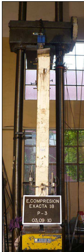
Foto 5. Modo de falla de la muestra. Falla por flexo-compresión en el extremo superior.
