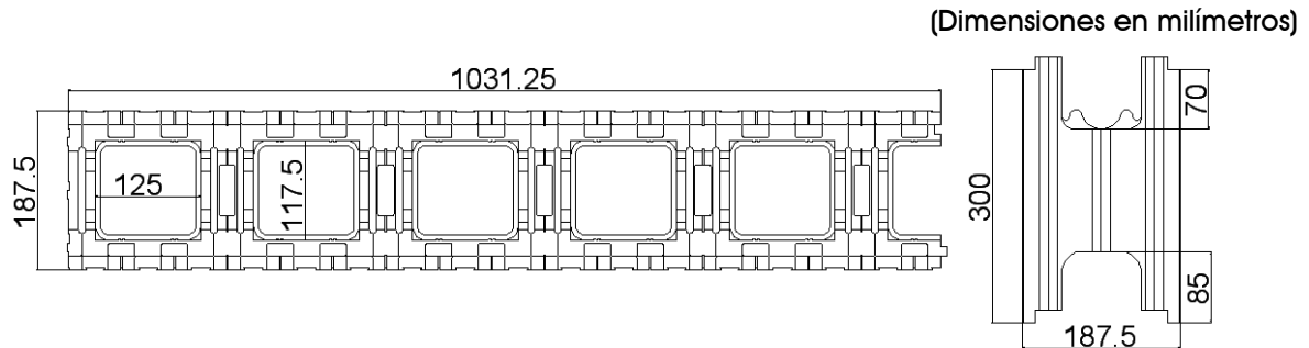
Figura 1: Esquema de unidad "Exacta 18".
