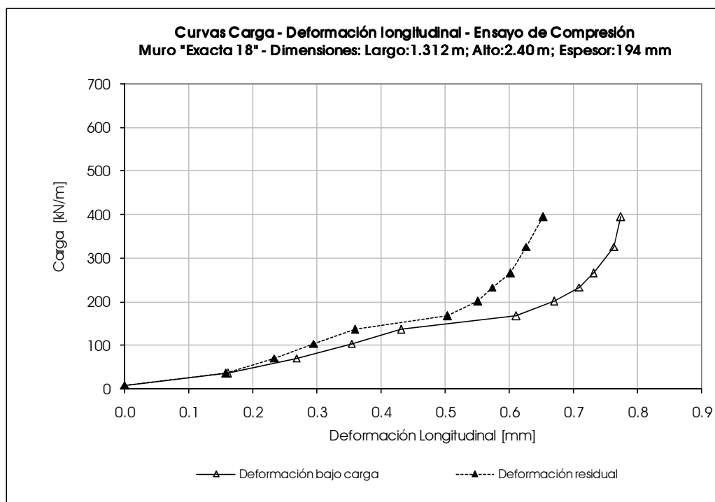
Gráfico 2. Curvas carga – deformación longitudinal (carga normalizada por el largo del muro). 4
